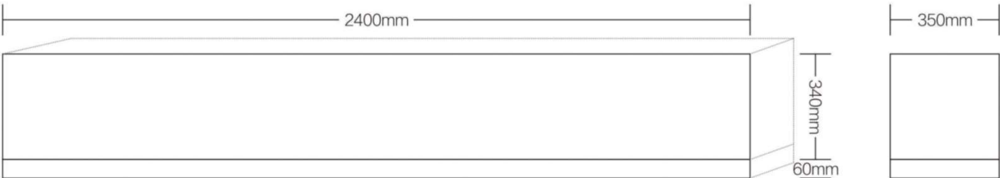
正视
