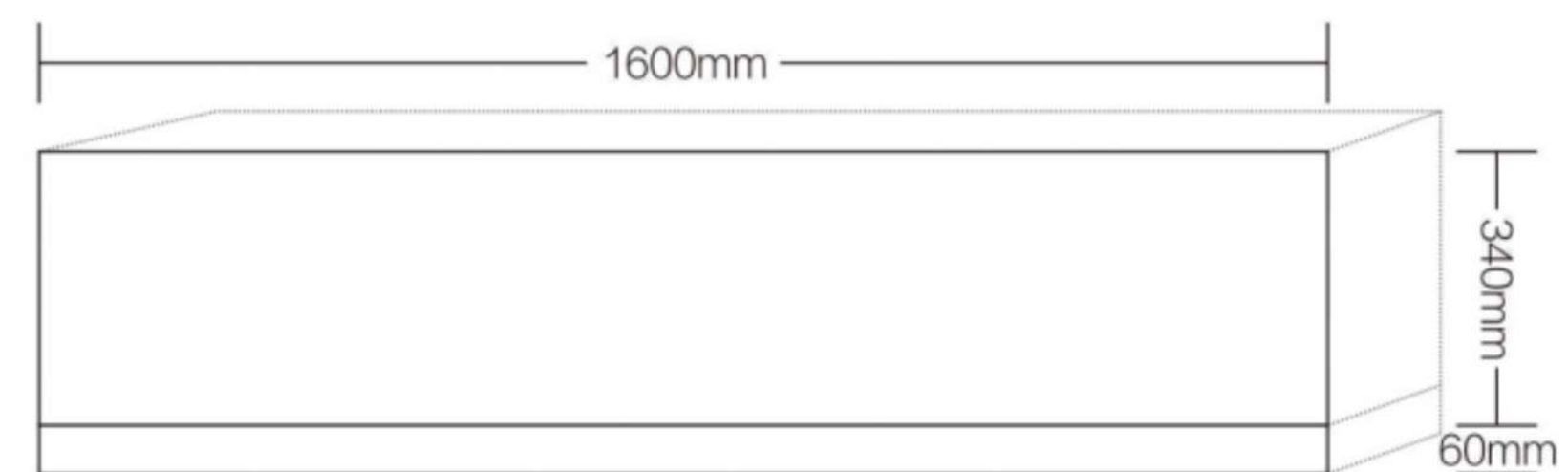
正视
